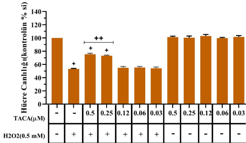
Şekil 3. GABA A reseptörler agonisti olan Trans-4-aminocrotonic acid'in (TACA) C6 glial hücrelerinde H 2 O 2 kaynaklı sitotoksosite sonrası hücre canlılığı üzerine etkisi. P<0.001 kontrol grubu ile karşılaştırıldığında; P<0,001, H 2 O 2 grubu karşılaştırıldığında.
